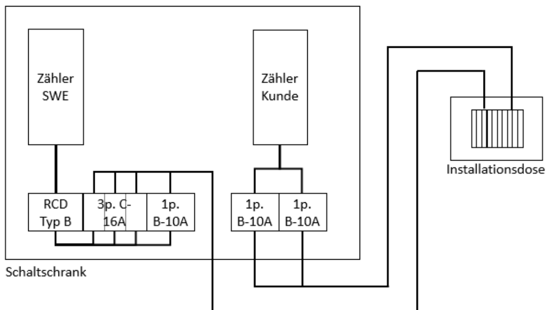
Abbildung 1: Schematische Darstellung Anschlüsse Strom
