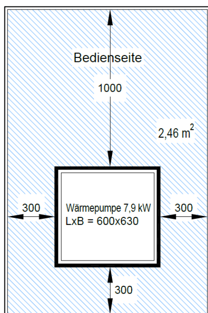
Abbildung 3: Platzbedarf Wärmepumpe Detail
