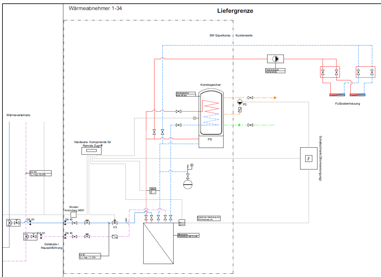
Abbildung 1: Schematische Darstellung der Systemgrenzen
